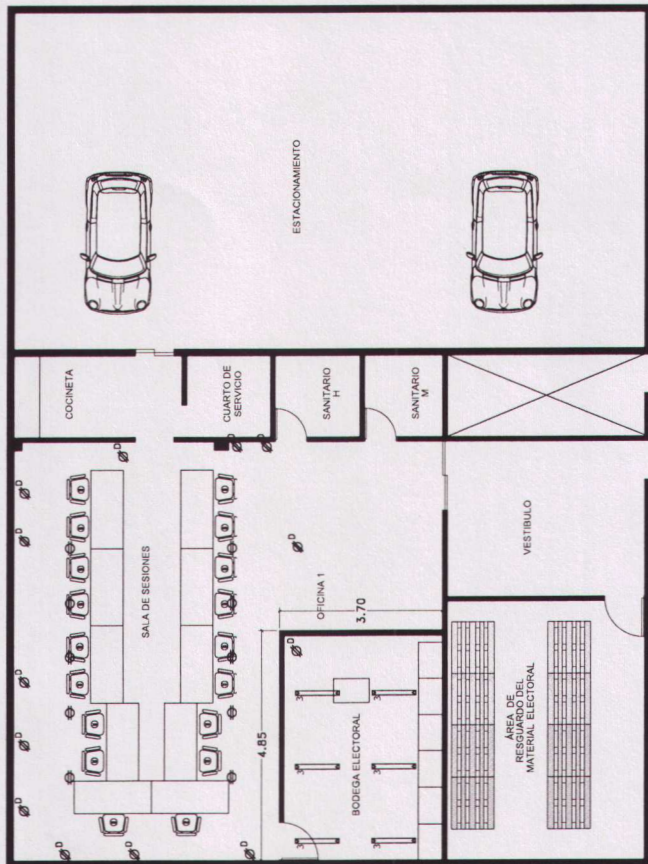
A PLANTA BAJA ESCALA S/N
